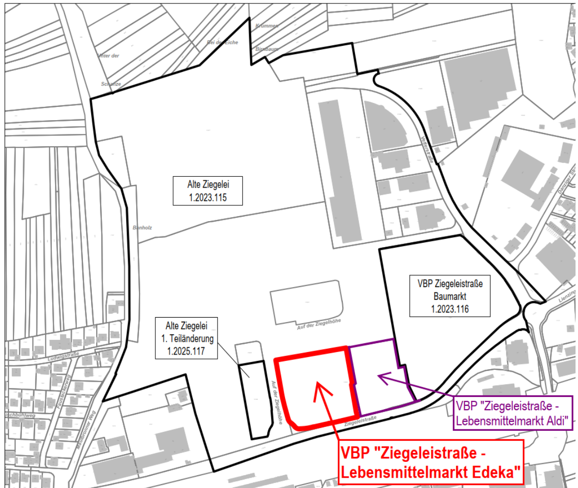
Übersichtsplan Abgrenzung Bebauungspläne
